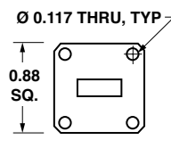
WR42 (UG-597/U)
