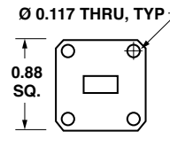
WR34 (UG-1530/U)
