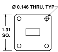
WR51 (MIL-F-3922/70-024)
