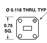
WR28 (UG-599/U)
