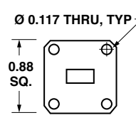
WR34 (UG-1530/U)
