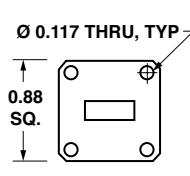
WR42 (UG-597/U)
